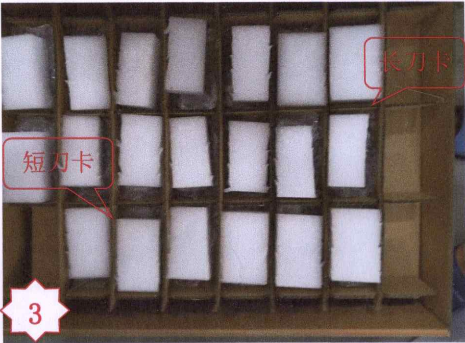
图三, 将 PA502 按照每层 120 个, 每箱三层的方式包装, 同时在底部和每层的顶部各放一块隔板, 共四块隔板。
